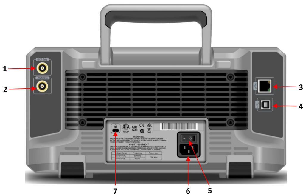
图 4-4 示波器后面板
