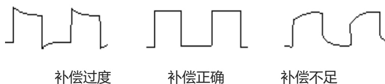
图 4-2 探头补偿校正
