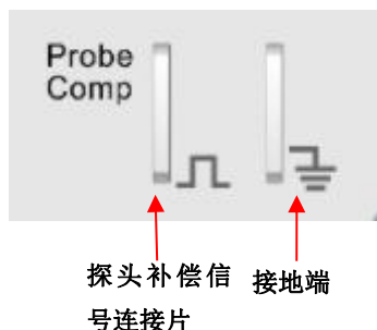
图 4-1 探头补偿信号连接片和接地端
