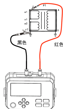
图10.2.3 二次绕组间绝缘电阻测试接线示意图
