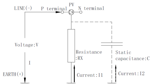
图9.3.2.1 PV Ω测量原理
