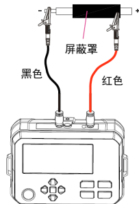
图10.1.1 常规两线测量接线示意图
