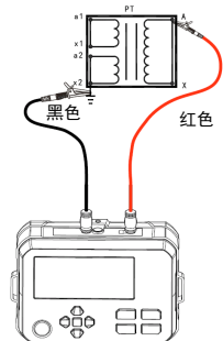
图10.2.1 一次绕组与二次绕组接地间绝缘电阻测试接线示意图
