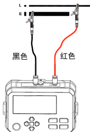
图9.3.3.2 电压测量接线示意图
