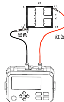
图10.2.2 一次绕组接地与二次绕组间绝缘电阻测试接线示意图
