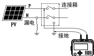
图10.3.1 P-N之间处于开路状态下测量
