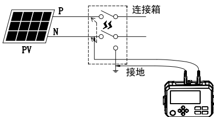
图10.3.2 P-N之间处于短路状态下测量
